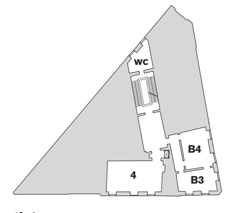
1° piano
